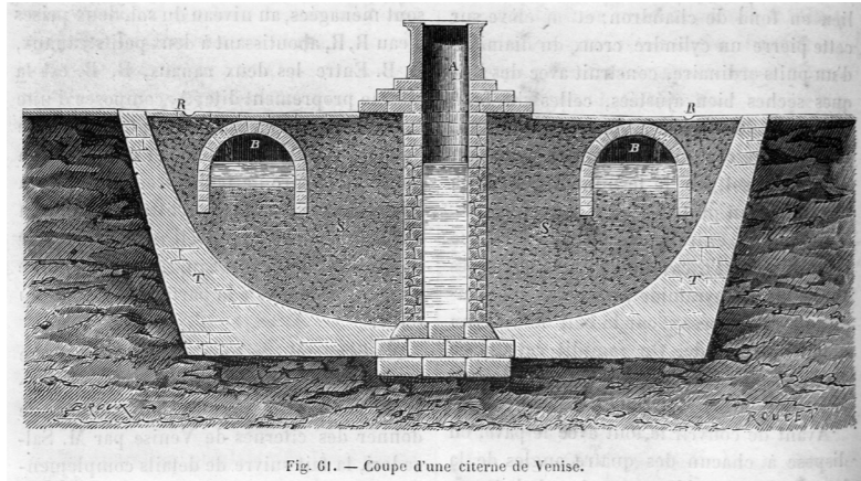
Fig. 61. — Coupe d'une citerne de Venise.
