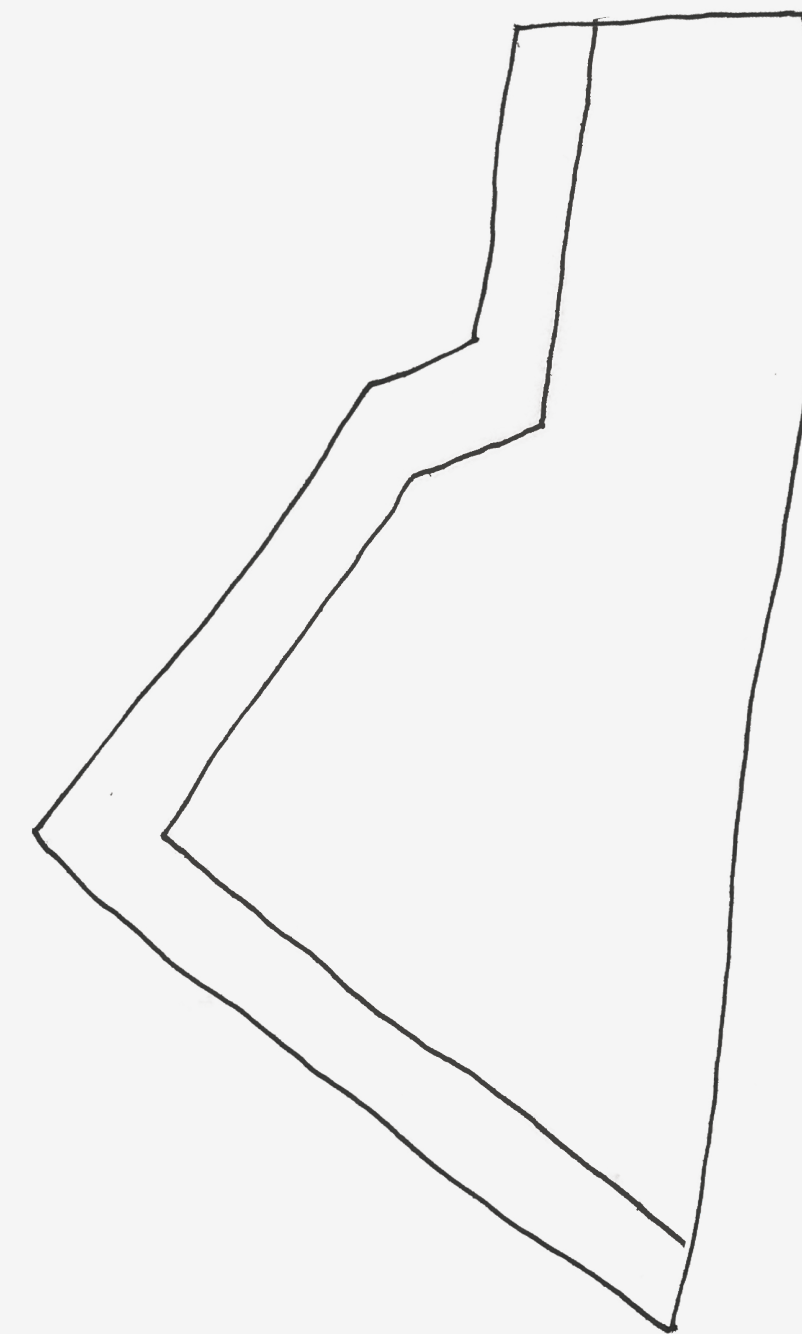
PLANTELAGUNER JORDDAMME 6 x 25 x 1,5 M. I ALT 31.500 M³
