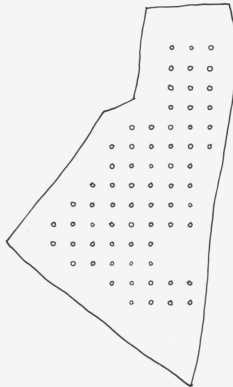
OPDRÆTSBASSINER 10M DIAMETER UDLAGT I GRID Å 50M. I ALT 69 BASSINER
