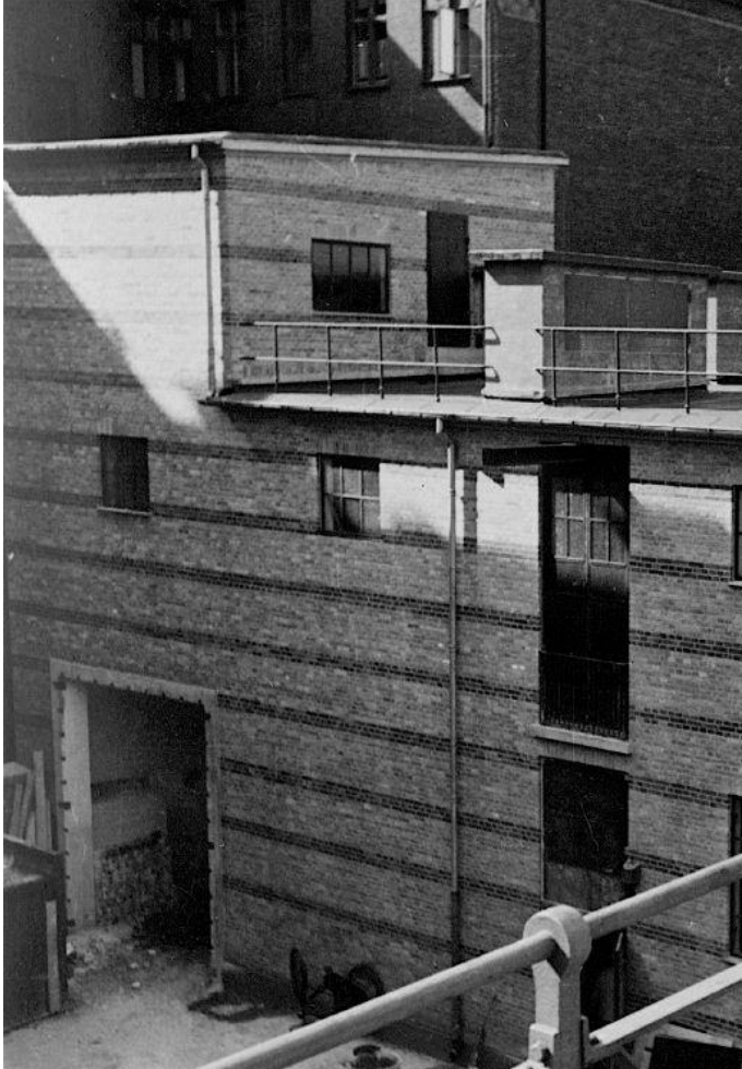
Østre Elektricitetsværk Udvidelse af højspændingsbygning 1943
