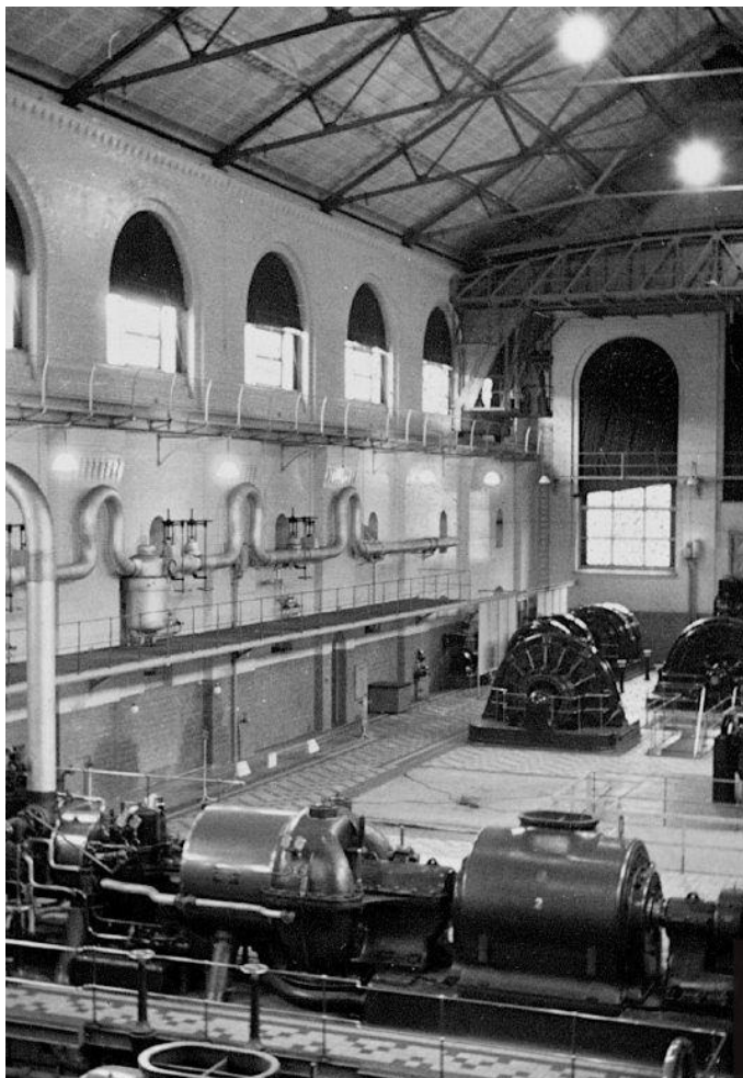
Østre Elektricitetsværk Maskinesal 1941
